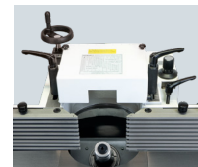
Fräsanschlag Typ 2601 mit Integralanschlagbacken
