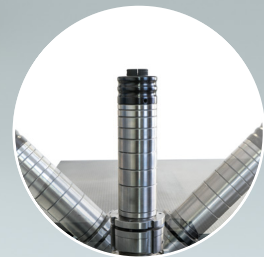
Starre oder schwenkbare Spindel (beidseitig 45,5°)
